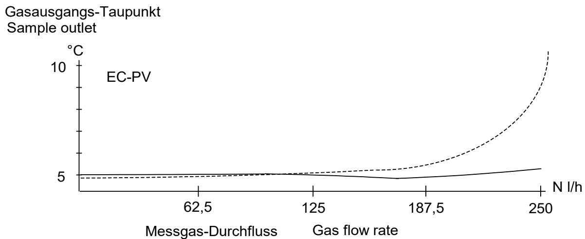
Abbildung 10: Messgas-Ausgangstaupunkt-Kennlinie
